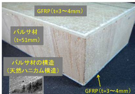
FRP サンドイッチ床版
