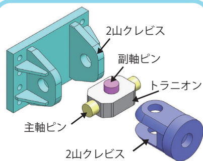
U-CLV の構造
