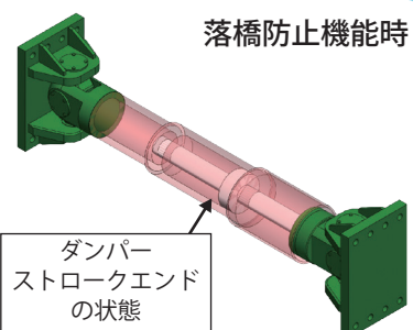
ダンパー本体が直接抵抗する構造
