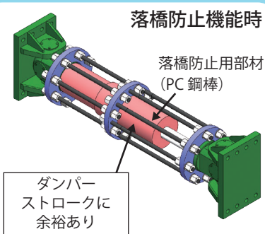
落橋防止用部材を増設した構造
