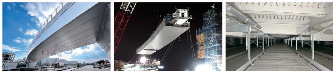
東扇島水江町線高架橋／神奈川県 新設橋に設置
