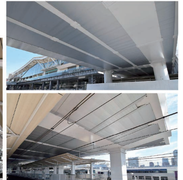
高輪ゲートウェイ駅／東京都 新設橋に設置
